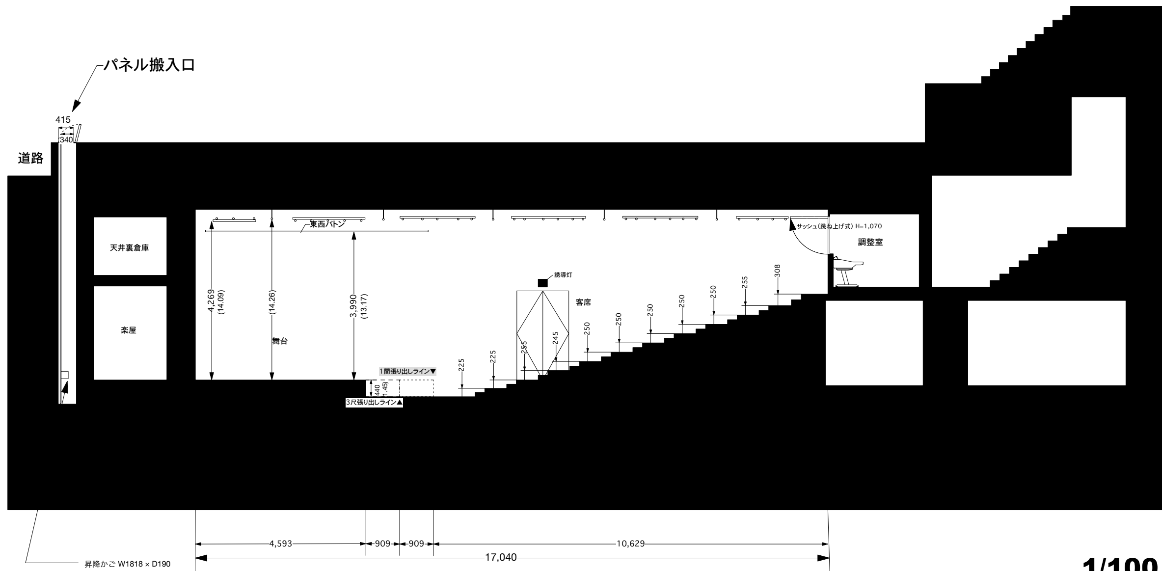
断面図
